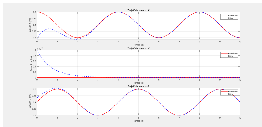
(a) Trajetórias da posição do punho ao longo do tempo
