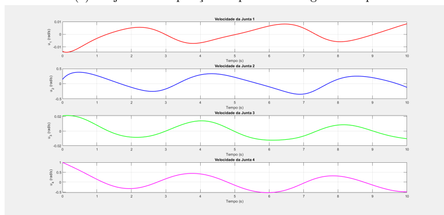
(b) Velocidades das 4 primeiras juntas
