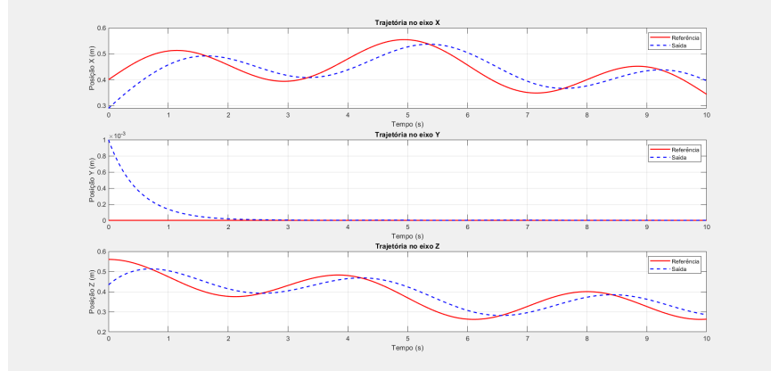
(a) Trajetórias da posição do punho ao longo do tempo
