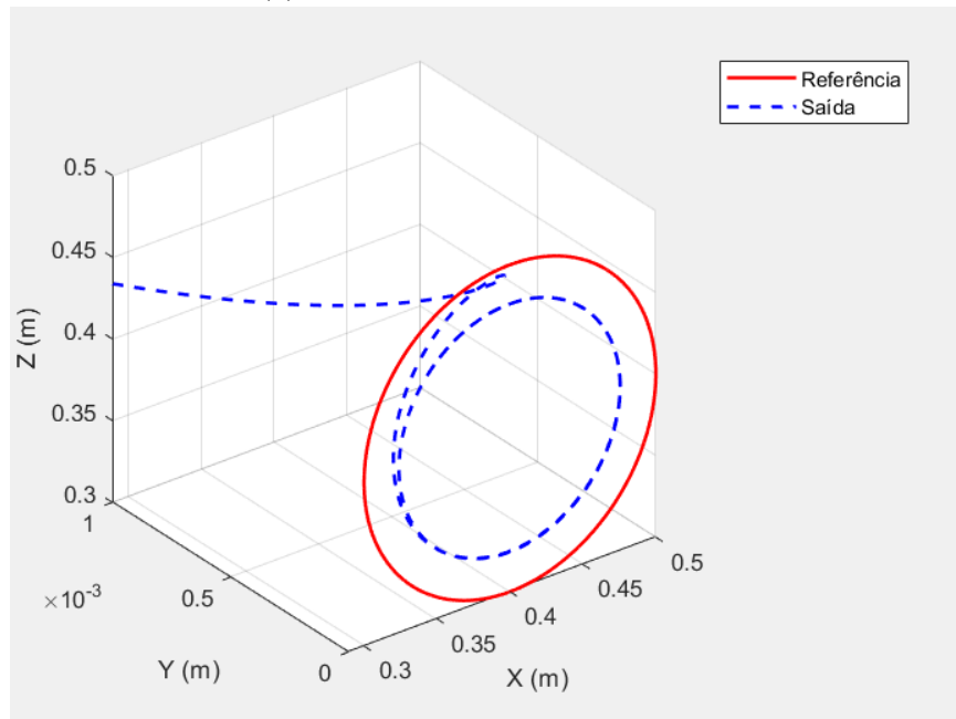
(c) Trajetória da posição do punho no espaço
